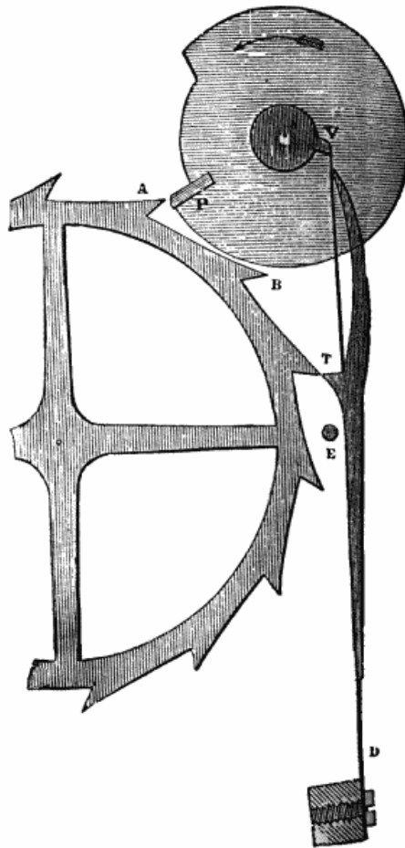
FIG. 76: CHRONOMETER ESCAPEMENT
